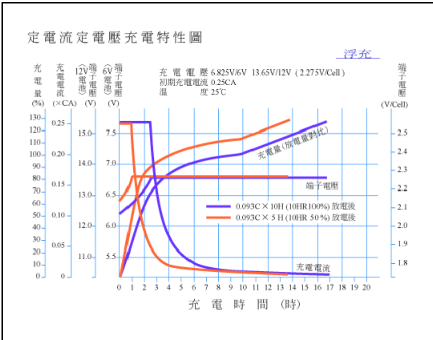
定電流定電壓充電特性圖
