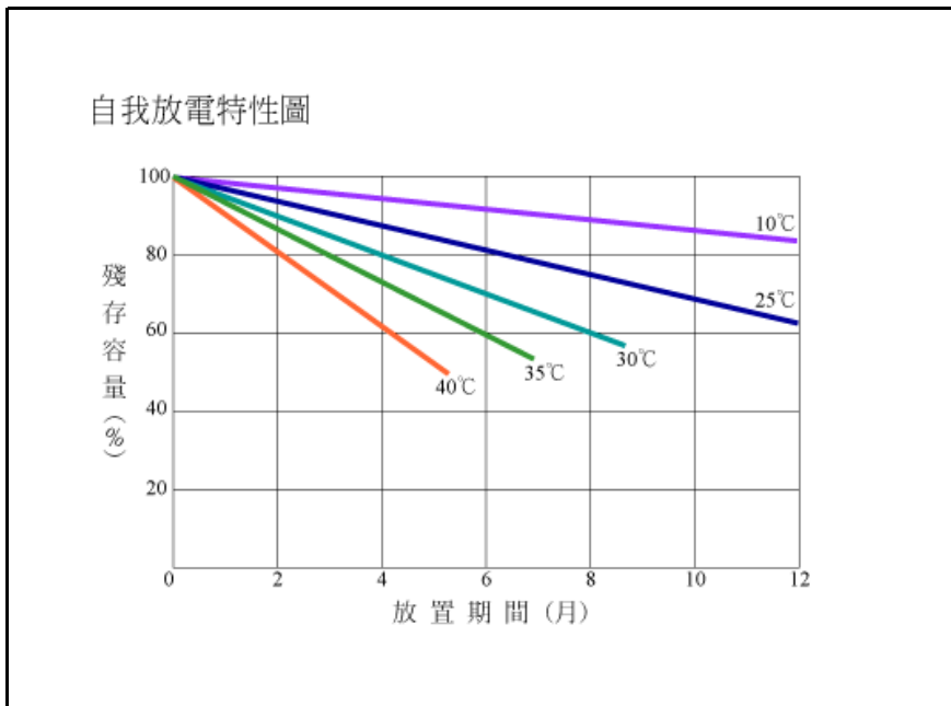
自我放電特性圖
