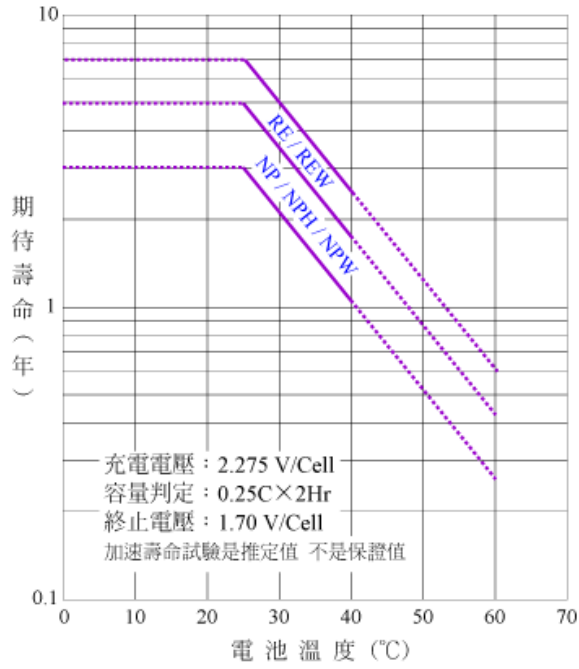
浮充期待壽命特性圖 (溫度 / 壽命)
